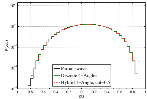
(d) 3000 mfp
