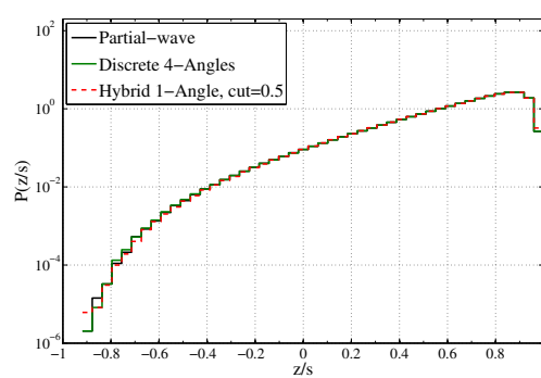
(d) 3000 mfp
