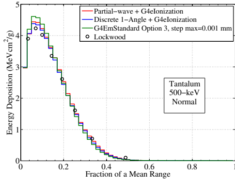
(a) 500-keV
